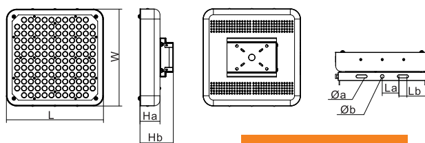
产品线条图
