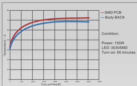
温升曲线
