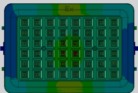
传导散热示意图（正面）
