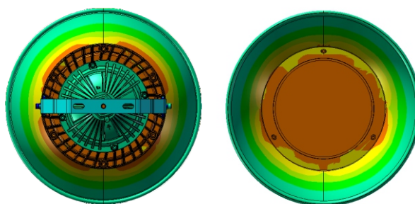
传导散热示意图
