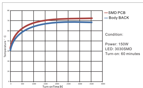
温升曲线
