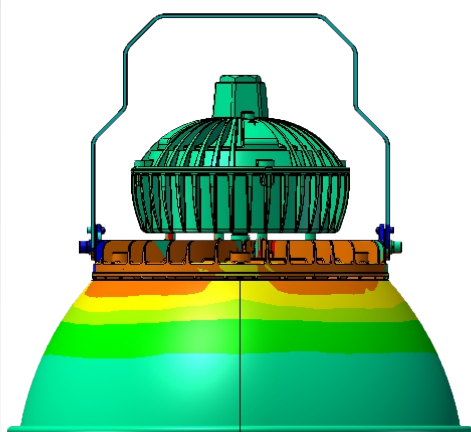
传导散热示意图
