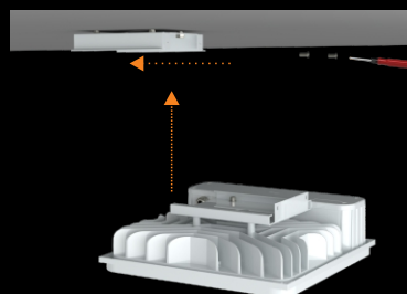
吸顶式安装 - 图2
