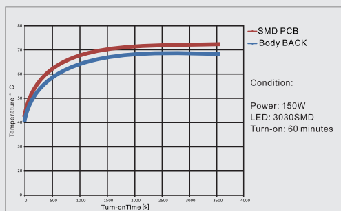
温升曲线
