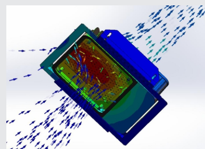
对流散热示意图
