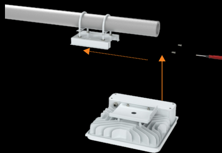
抱管式安装 - 图2
