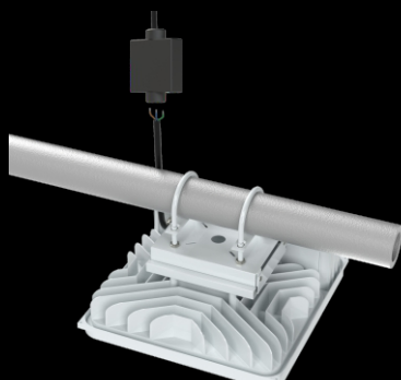
抱管式安装 - 图3
