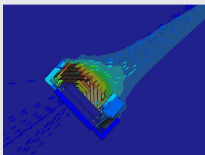
灯具热量对空气的影响
