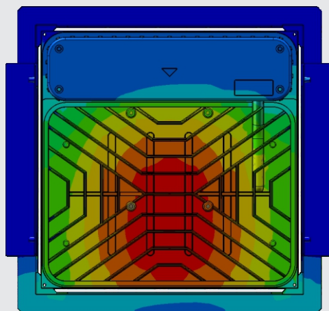
传导散热示意图（背面）
