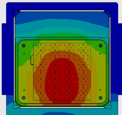
传导散热示意图（正面）
