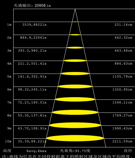
150W 平均照度图
