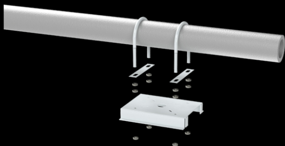
抱管式安装 - 图1
