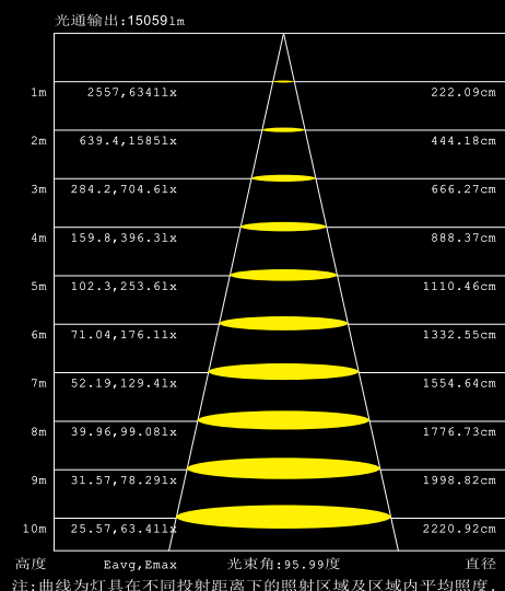
100W 平均照度图
