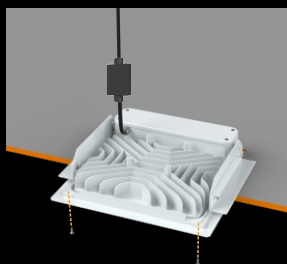
嵌入式安装 - 图3
