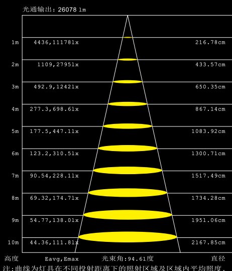
200W 平均照度图
