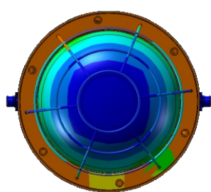
传导散热示意图（正面）
