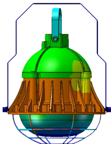
传导散热示意图（侧面）
